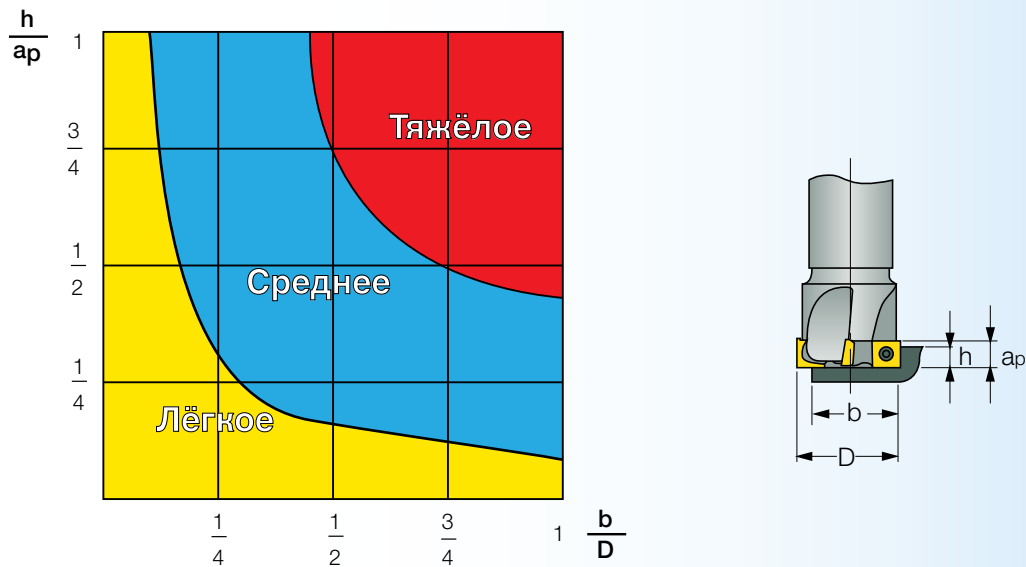
Рис. 1. Области нагружения зуба
